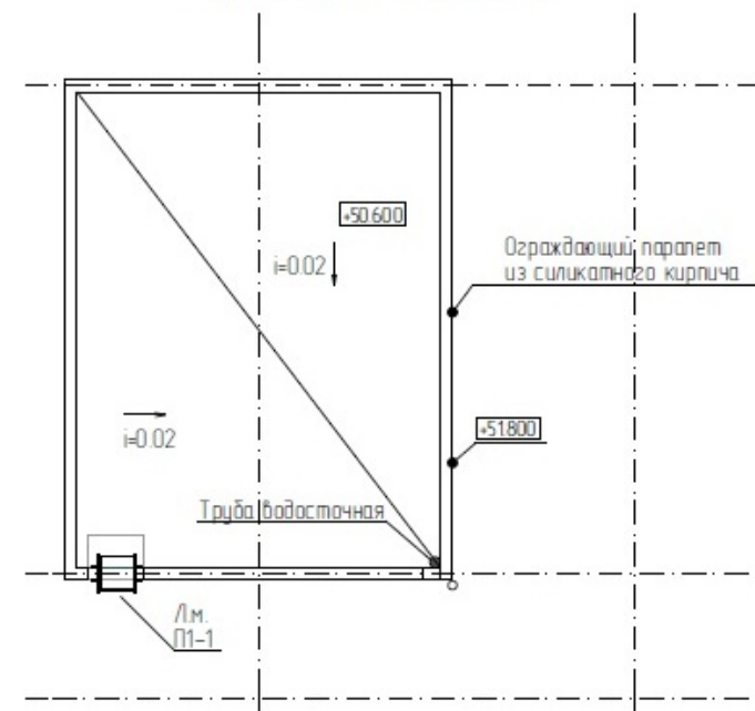
Фрагмент кровли на отметке +51.900
